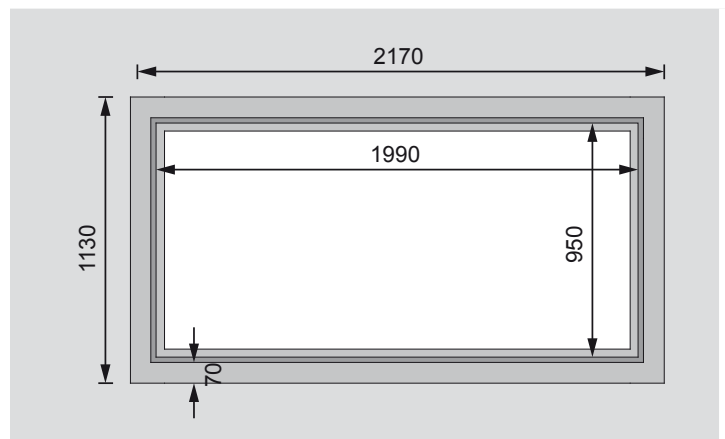
Draufsicht (in mm)
